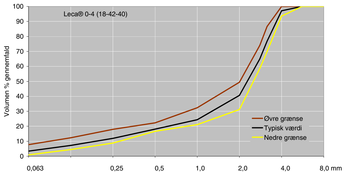
Vejledende sigtekurve omregnet til volumen gennemfald
